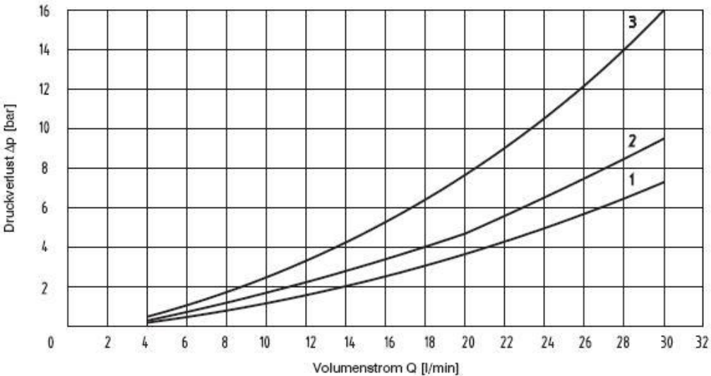
\Delta p -Q 曲线测量值 v = 32 \text{ mm}^2/\text{s} 来自流量中的压力损失 \Delta p
