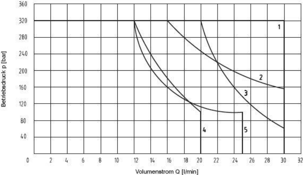
p-Q 曲线测量值 v = 32 \text{ mm}^2/\text{s} 最高限额，方向阀液压动力传输
